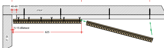
Schéma de pose et travail avec des découpes de panneaux
