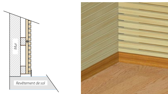
Détail de la finition par un tasseau
