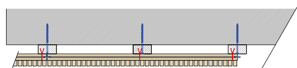
Agrafes dans la rainure avec la grille de renfort (Marilyn 4-12)
